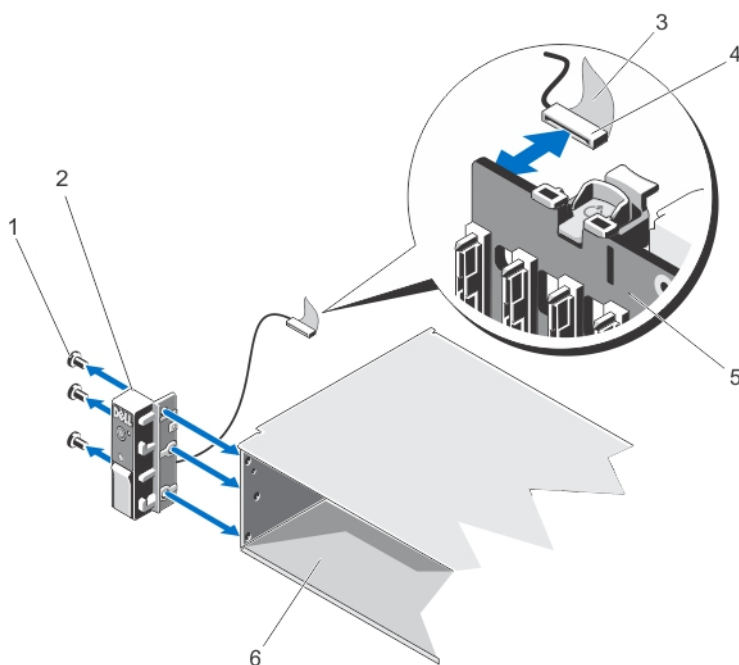
图 43: 卸下和安装控制面板
