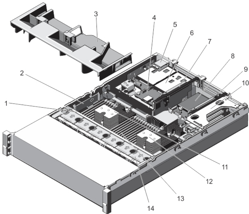
图 9: 系统内部组件
