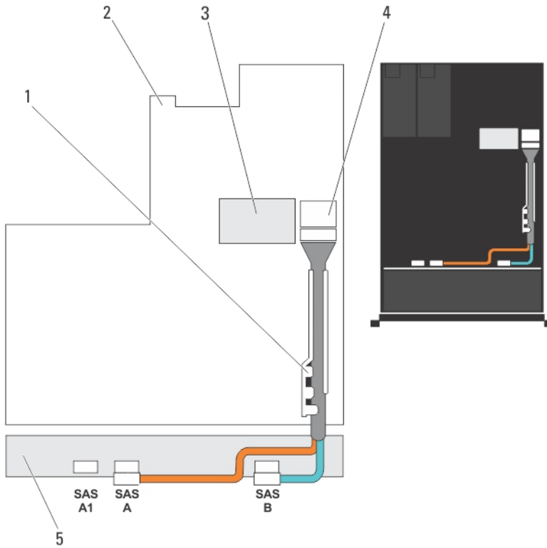
图 42: 布线图—3.5 英寸 (x12) SAS/SATA 背板
