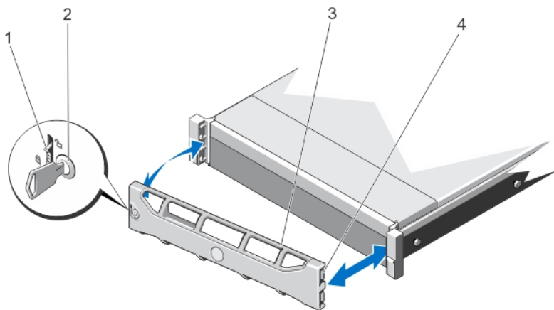
图 7: 卸下和安装前挡板
