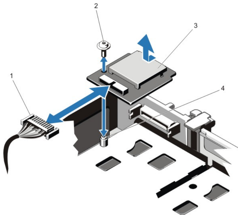
图 31: 卸下和安装 vFlash 介质单元
