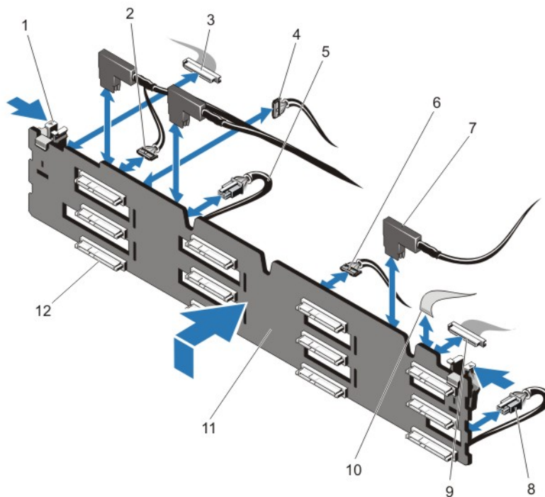
图 41: 卸下和安装 3.5 英寸 (x12) SAS/SATA 背板
